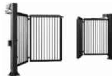
Remplissage en panneaux VEGA 2D Super (soudés à la structure)
