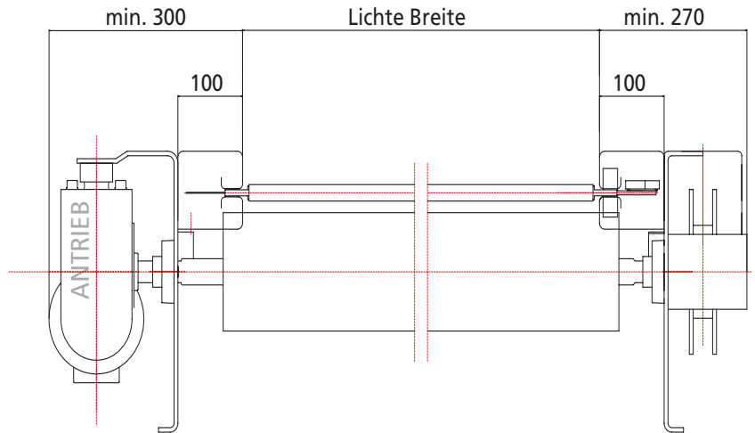
Schnellaufmotor mit Gegengewicht (siehe Tabelle)
