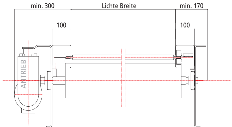
Schnellaufmotor ohne Gegengewicht (siehe Tabelle)
